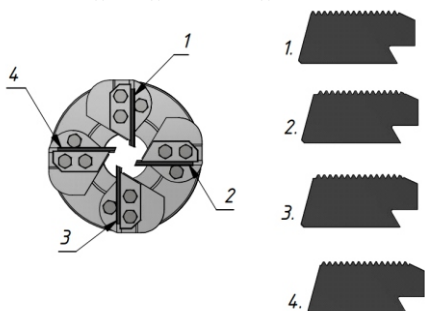
Рис.1 Резьбонарезная головка
